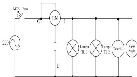
Gambar 7 Pengukuran terhadap Lampu TL, Tv & Kipas angin tanpa alat penghemat daya
