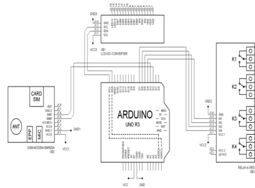
Gambar 2 Skema rangkaian
