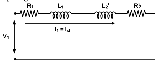
Gambar 3. Rangkaian ekivalen motor induksi 3-fasa perfasa saat start dengan analisa transien
