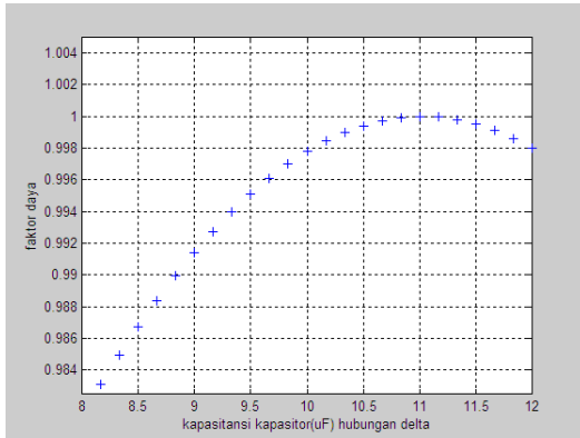
Gambar 5. Hubungan perubahan nilai kapasitansi kapasitor terhadap faktor daya motor
