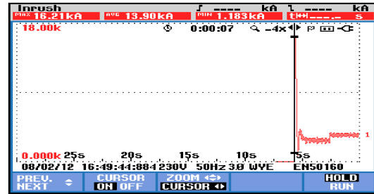
Gambar 8. Arus start motor saat menggunakan kapasitor 10 uF
