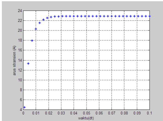
Gambar 11. Hubungan arus transien start (transien) motor induksi terhadap waktu
