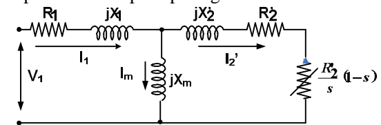
Gambar 1. Rangkaian ekivalen motor induksi 3-fasa perfasa
