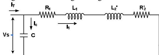
Gambar 13. Rangkaian ekivalen motor saat distar menggunakan kapasitor
