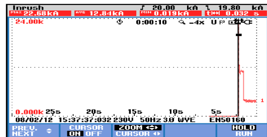
Gambar 9. Arus start motor saat menggunakan kapasitor 60 uF
