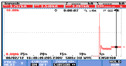
Gambar 7. Arus yang melewati kumparan motor
